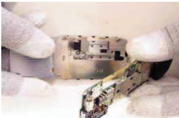
21) Remove the PWB.
