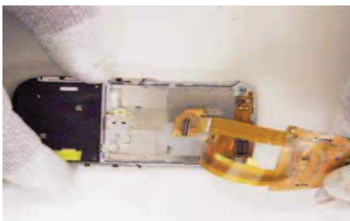
23) Remove the UI Flex.
